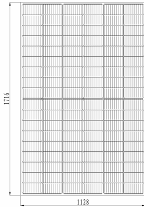
正面视图
