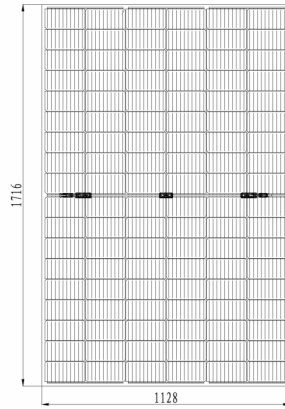
背面视图
